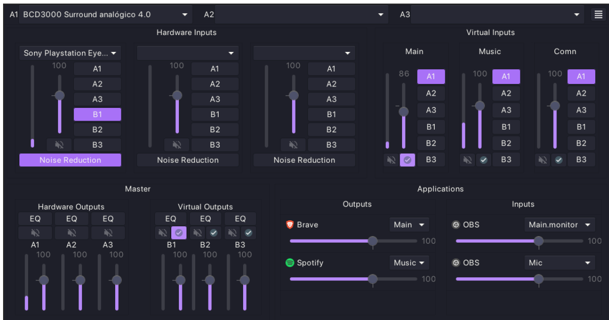
Figura 24 – Segunda versão da aplicação, a interface ainda era similar a do Voicemeeter, porém já incluía controles para cada aplicação
