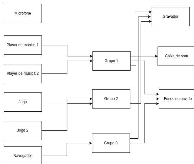
Figura 21 – Uma possível rota do áudio das aplicações em um sistema quando se utiliza grupos
