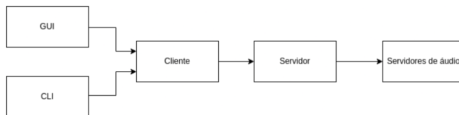
Figura 22 – Arquitetura do sistema, com uma clara separação entre clientes e servidor
